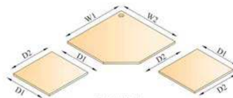
PENTAGON TOP W1=900,1050 W2=900,1050 D1=450,500,600,750 D2=450,500,600,750
